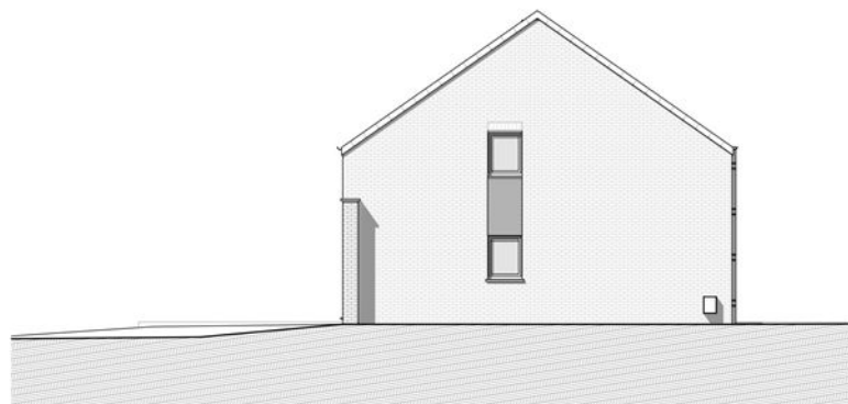
Façade droite - lot 5 -
