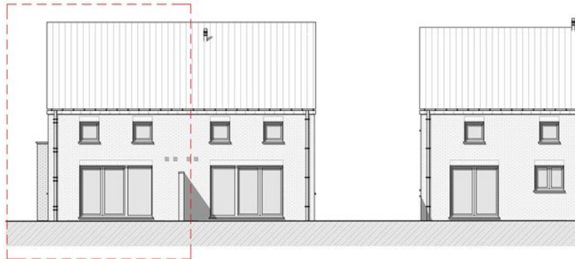
Façade arrière - lot 5 -
