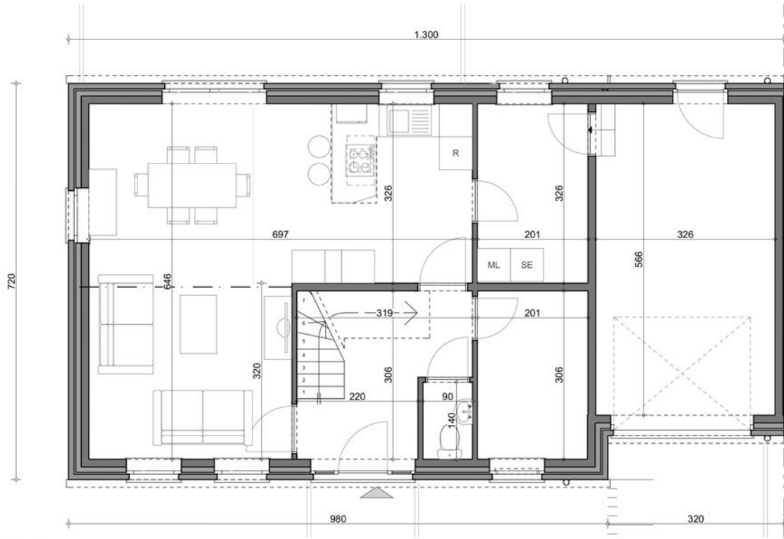
Plan rez-de-chaussée - lot n° 2 -
