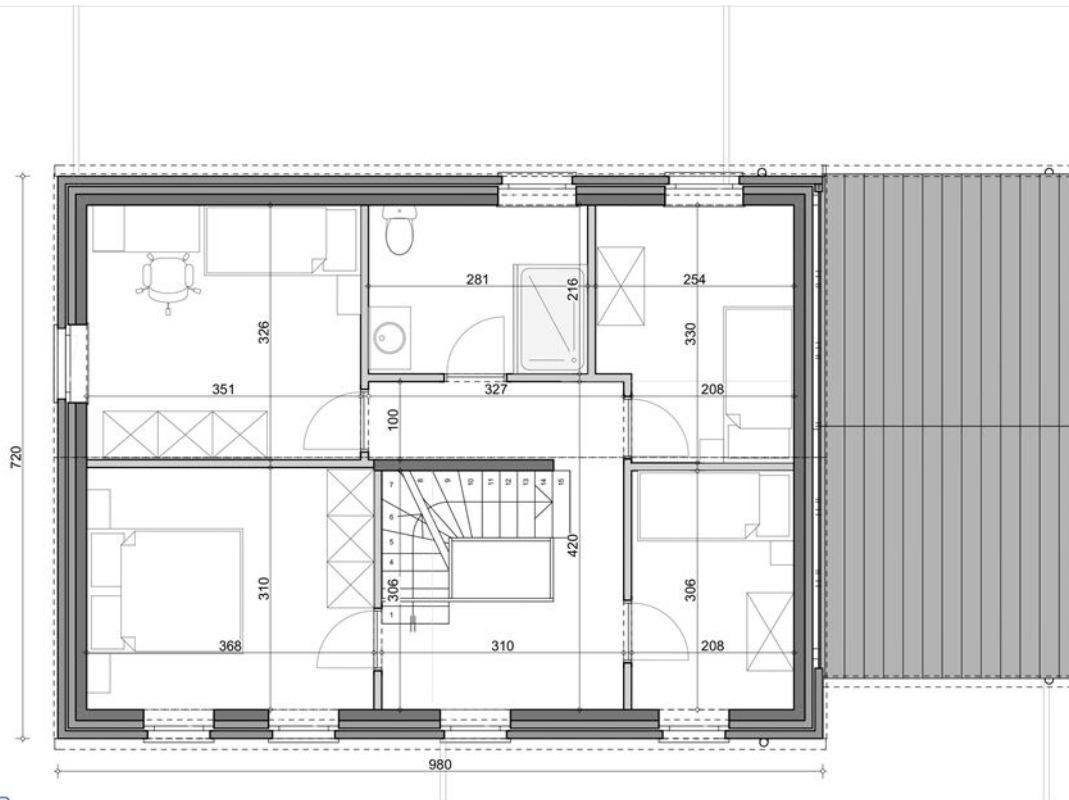
Plan étage - lot n° 2 -
