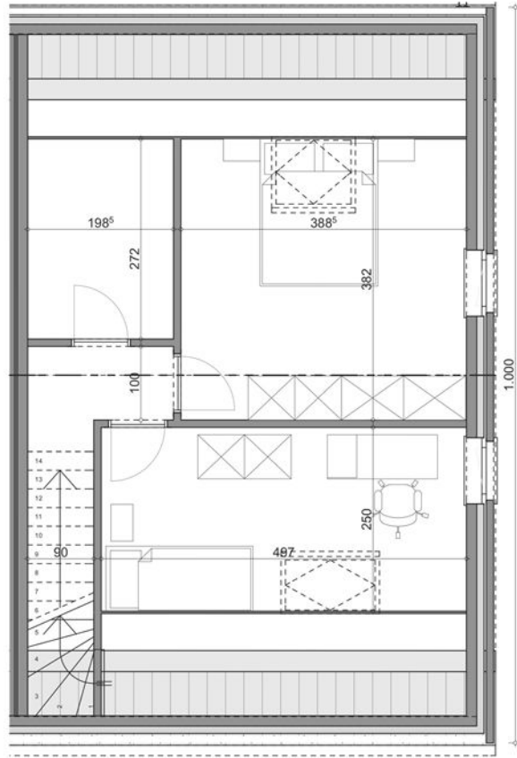
Plan 1er étage - Lot n°5 -
