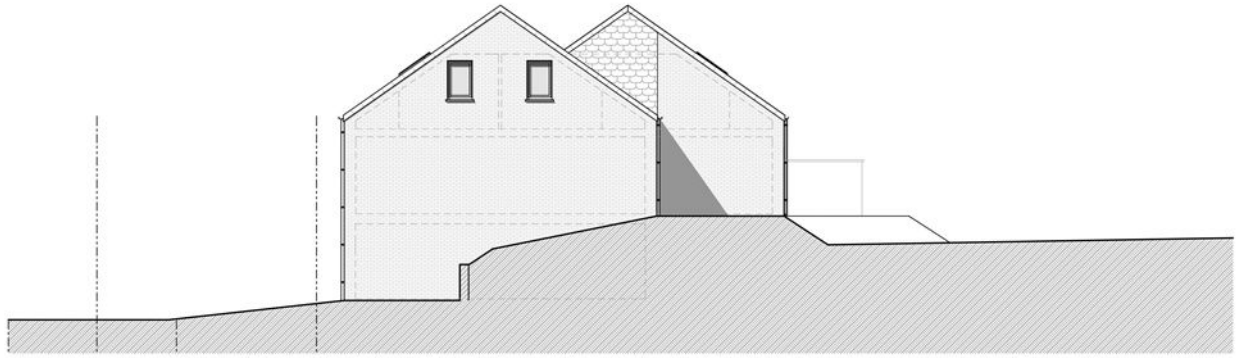
Façade droite - Lot n° 5 -
