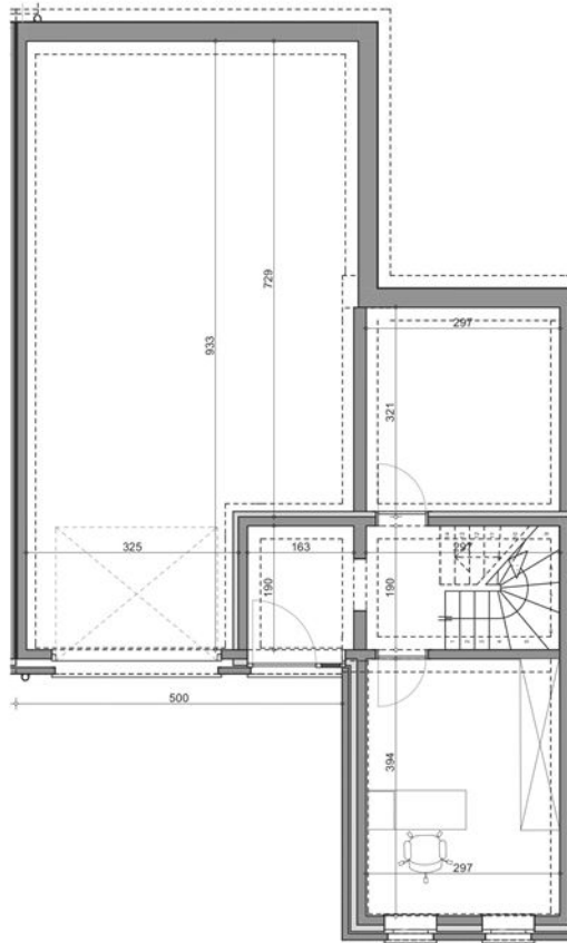
Plan sous-sol - Lot n° 4 -
