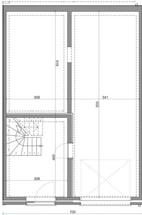
Plan sous-sol - Lot n° 2 -
