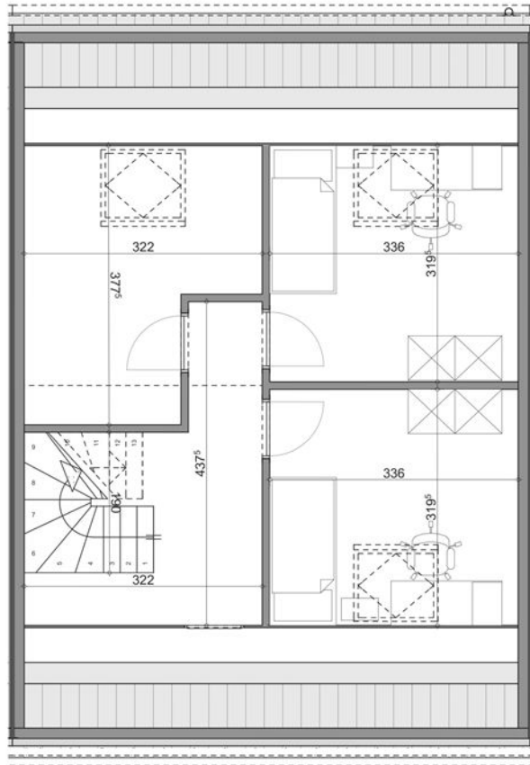
Plan 1er étage - Lot n°2 -
