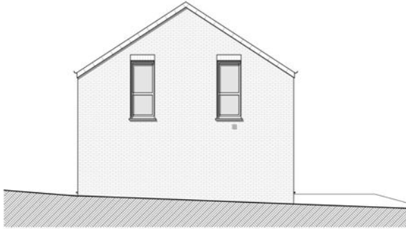
Façade droite - lot n° 2 -
