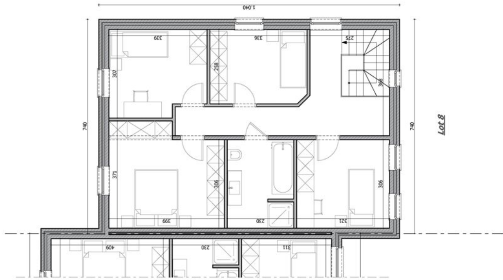
Plan étage Lot n°8
