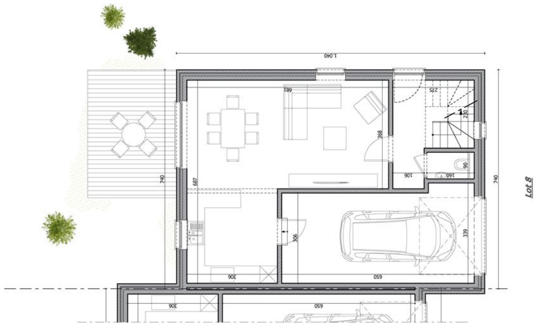
Plan rez Lot n°8
