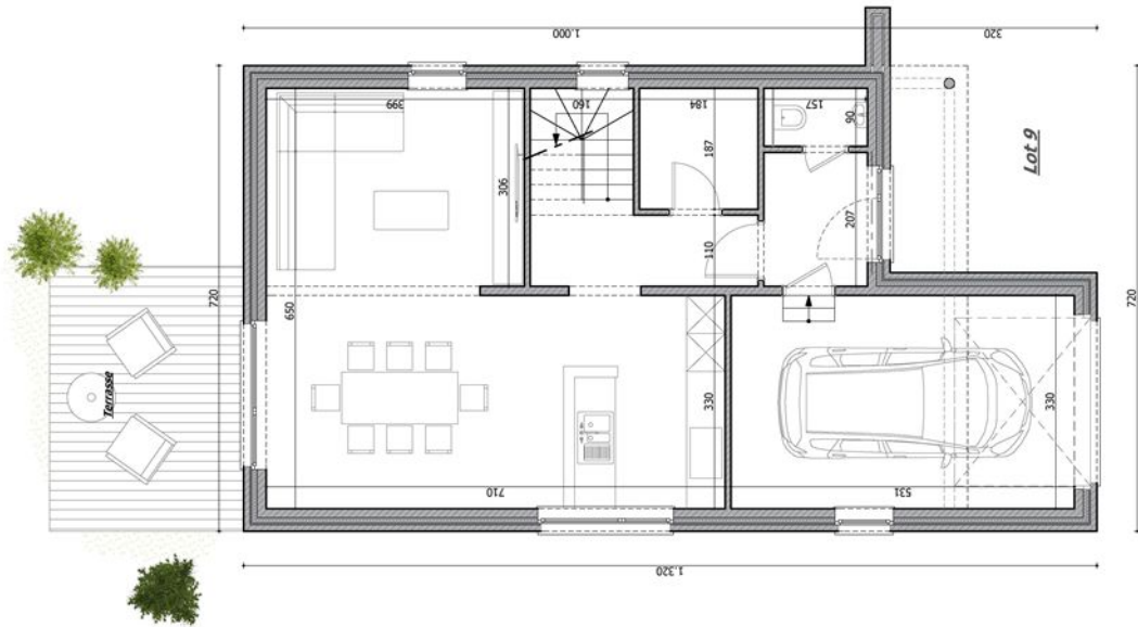
Plan rez Lot n°9
