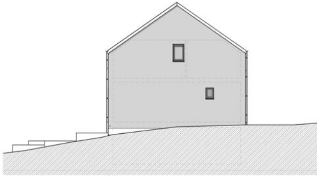
Façade Droite
