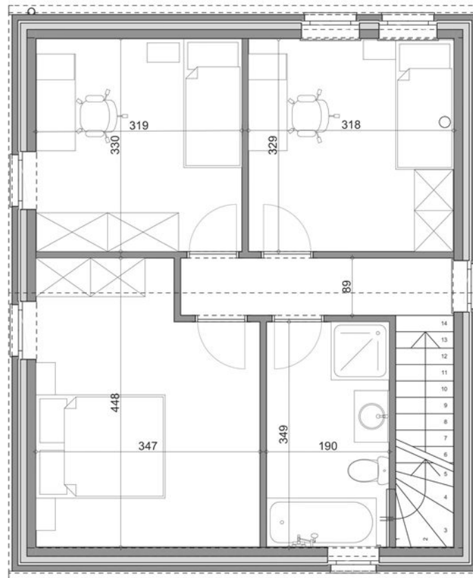
Plan Etage
