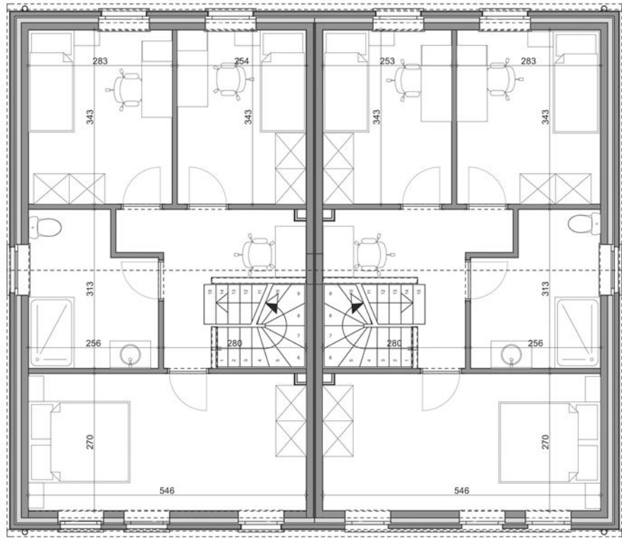
Plan étage - lot n° 1 -
