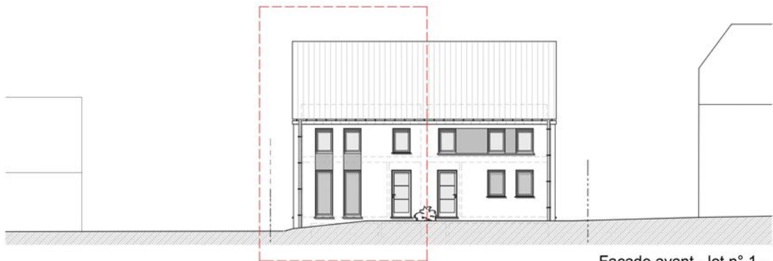
Façade avant - lot n° 1 -
