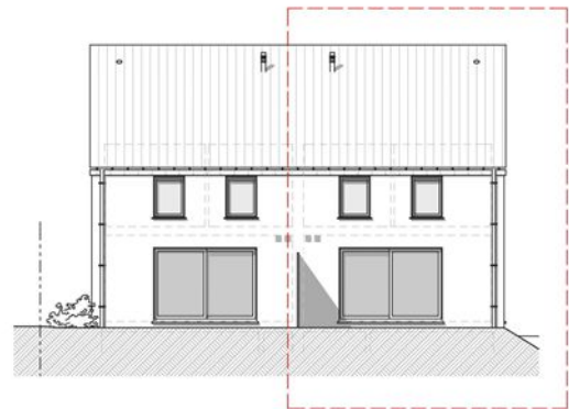
Façade arrière - lot n° 1 -
