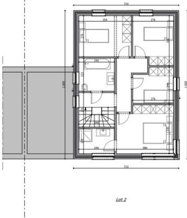
Plan étage Lot n°2
