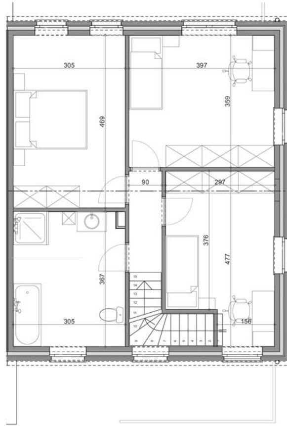
Plan 1er étage - Lot n° 2 -
