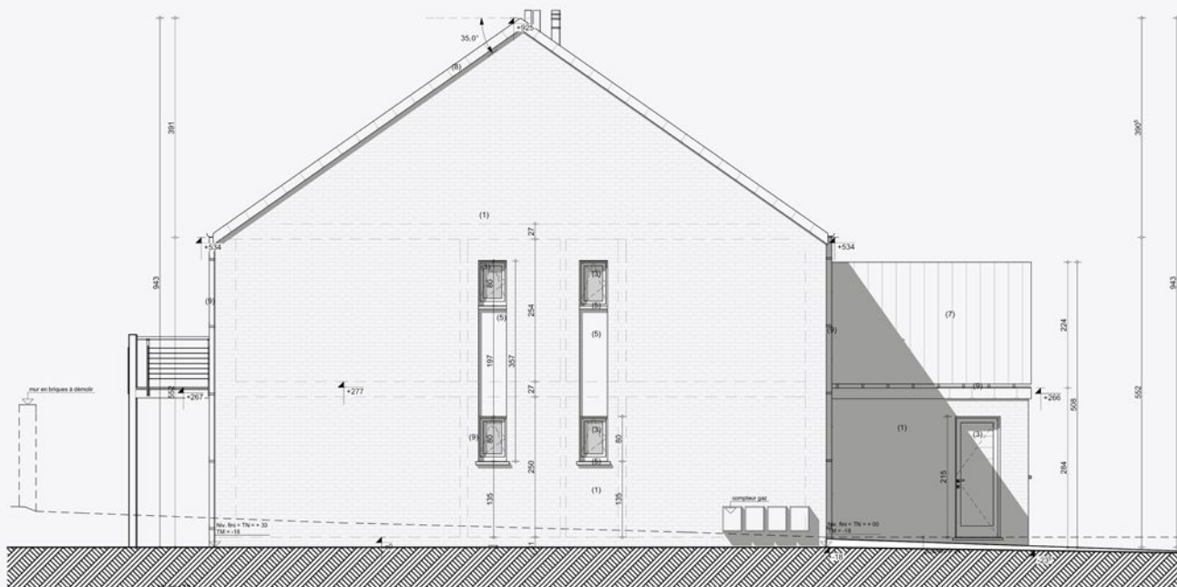
Pignon gauche
