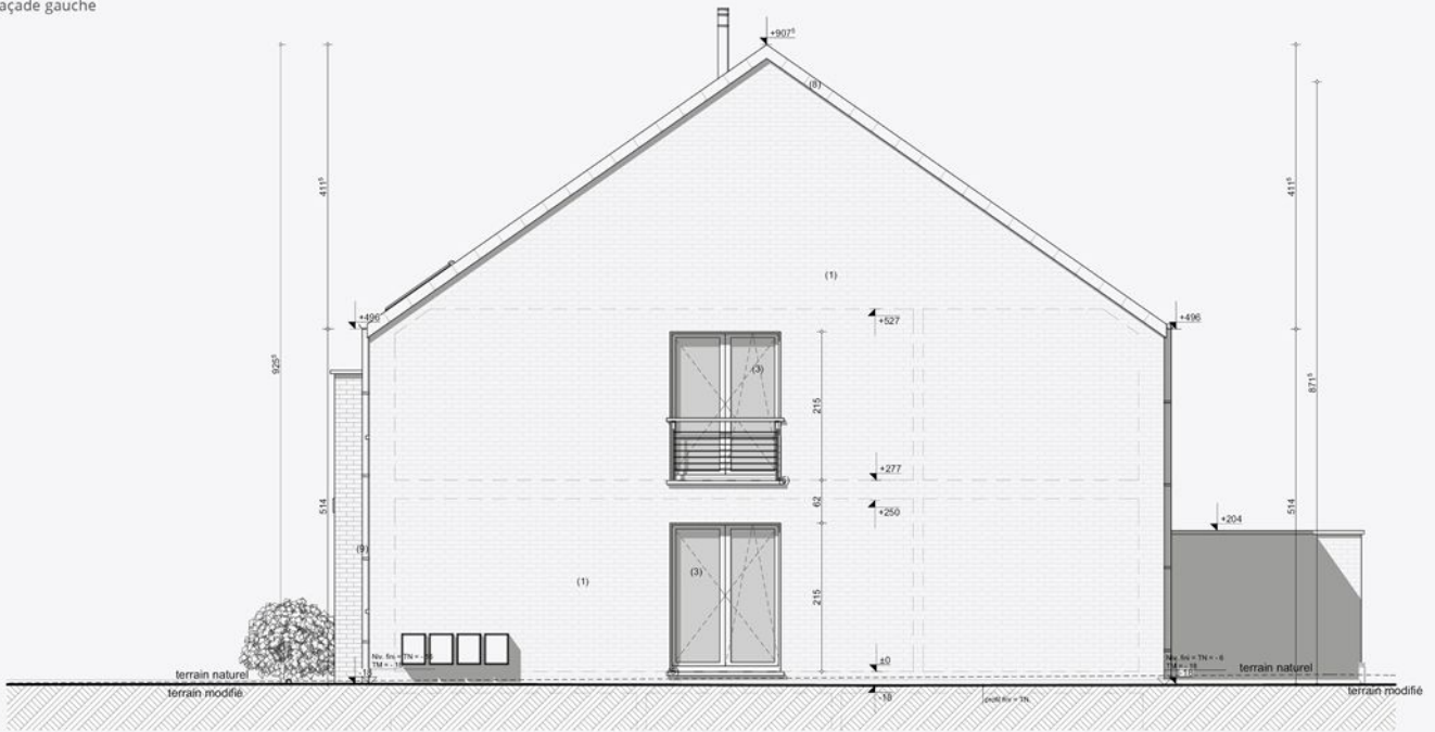
Façade gauche
