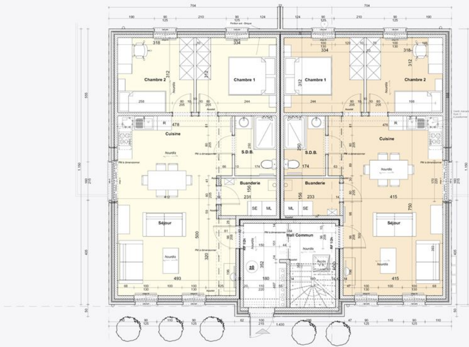
Rez-de-chaussée
