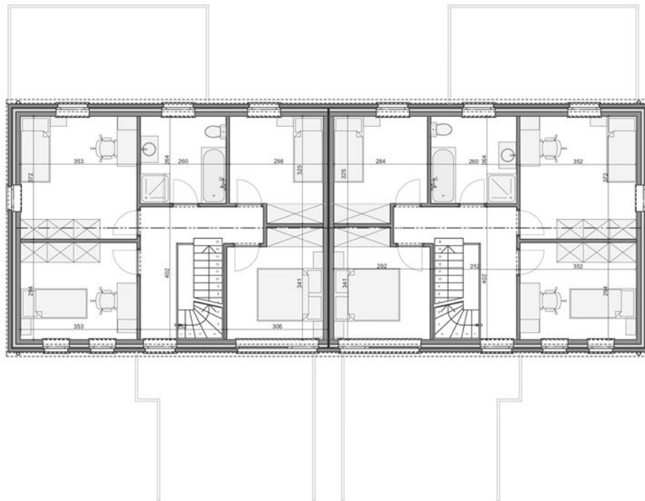
Plan 1er étage - Lot n° 1 -
