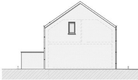
Façade gauche - Lot n° 1 -
