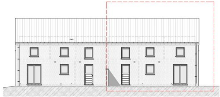
Façade arrière - Lot n° 1 -
