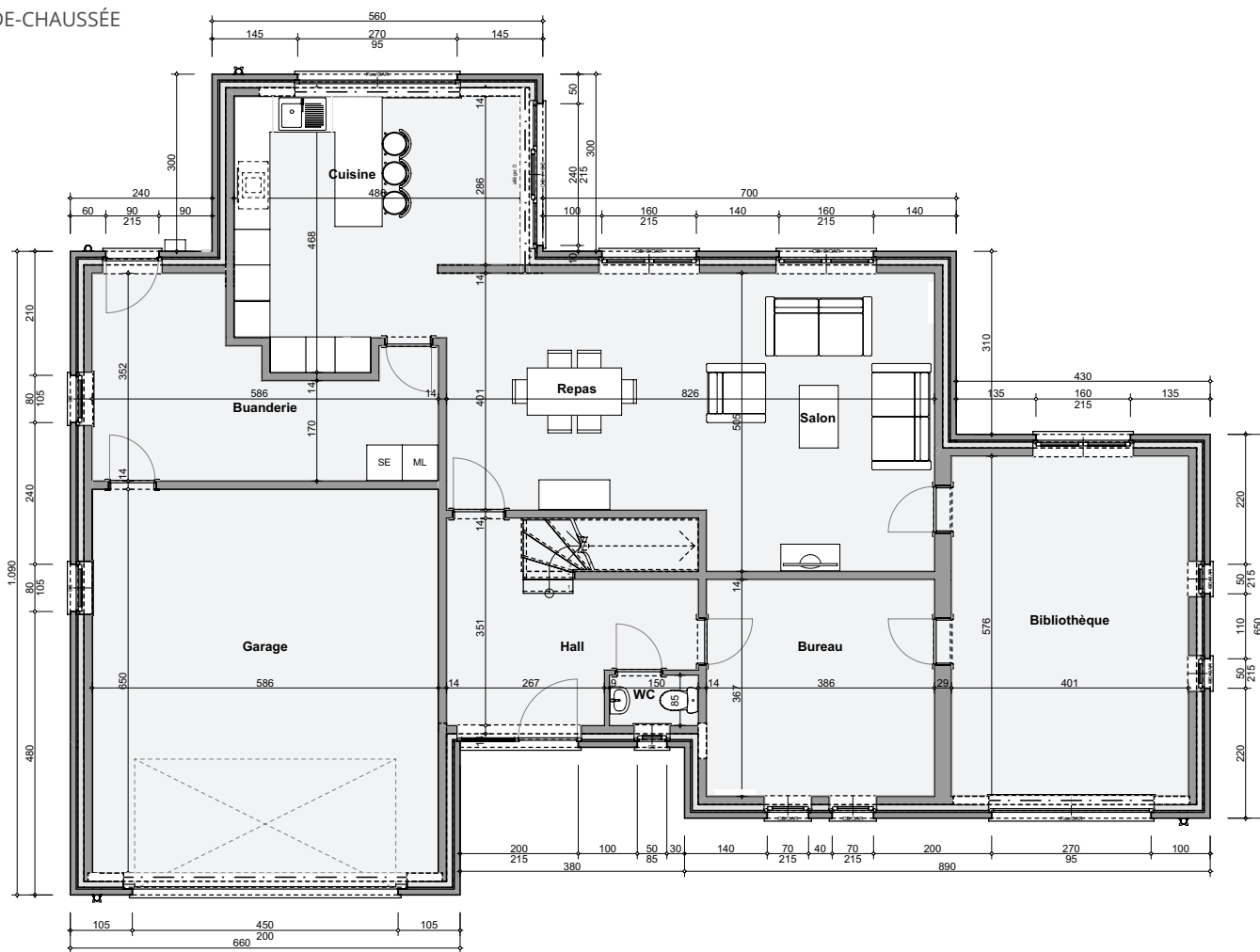
REZ-DE-CHAUSSÉE
